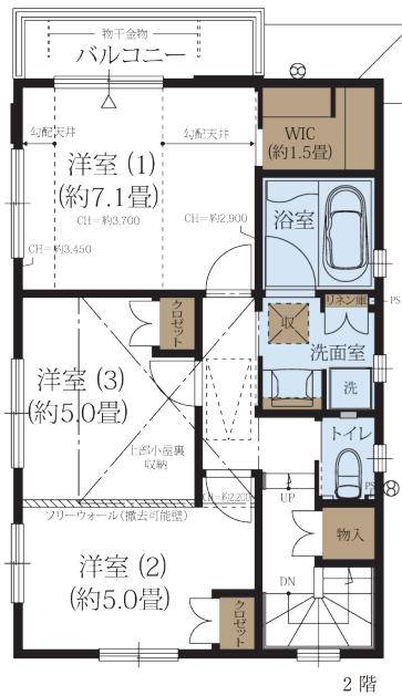
2階
