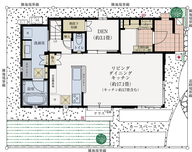
■1階平面図
