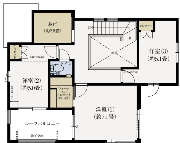
■2階平面図
