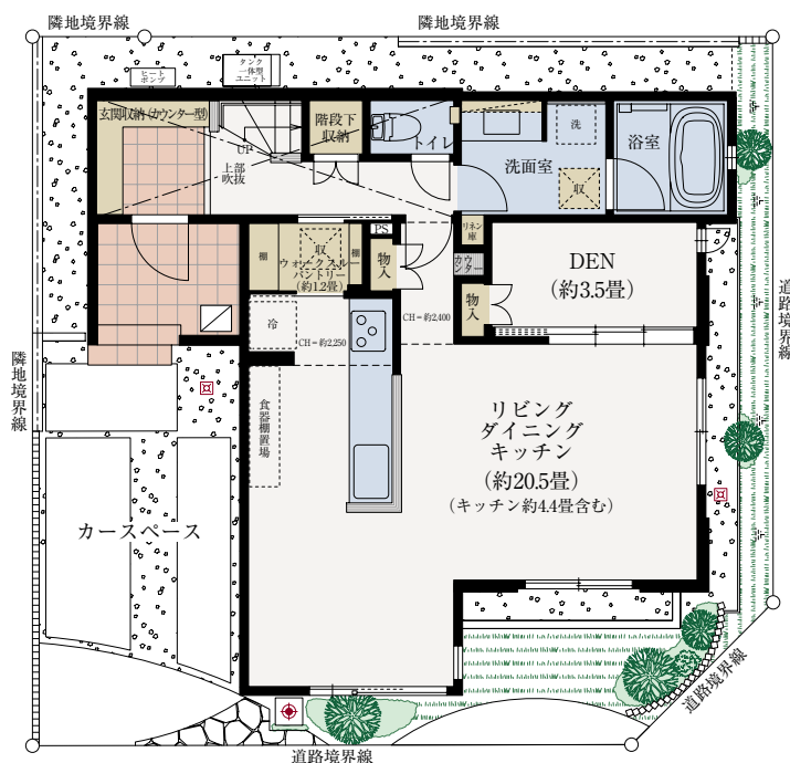
■1階平面図
