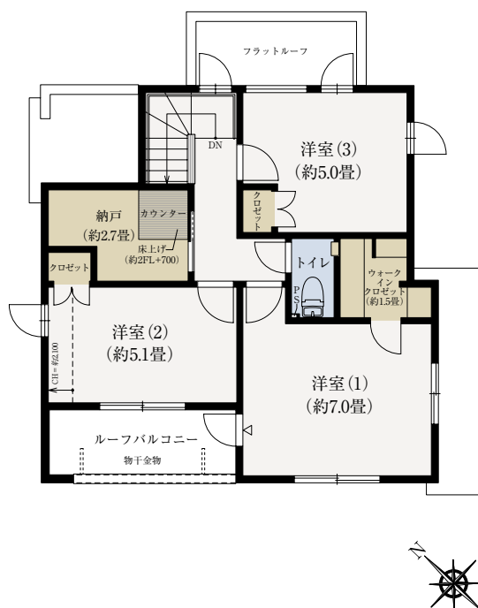
■2階平面図
