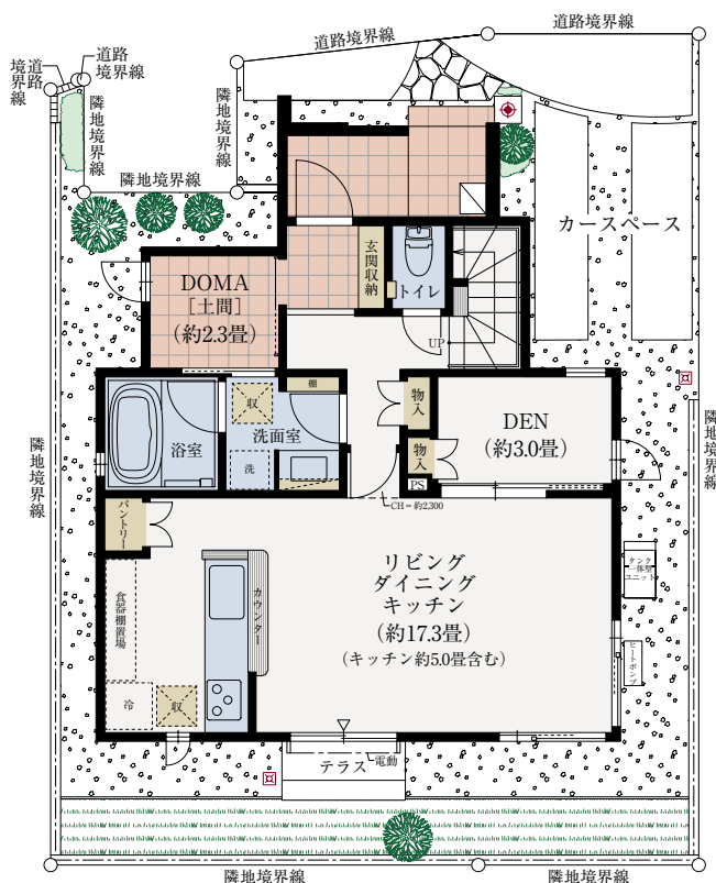
■1階平面図
