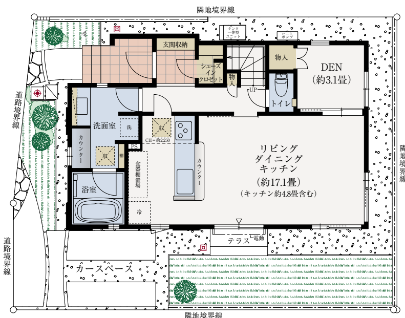
■1階平面図
