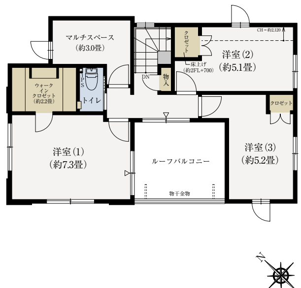
■2階平面図
