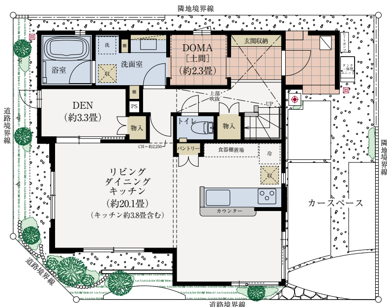
■1階平面図
