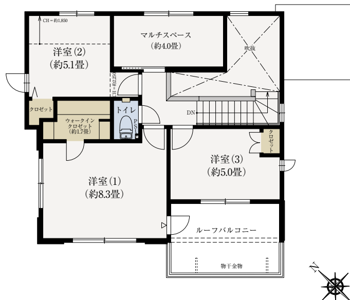
■2階平面図
