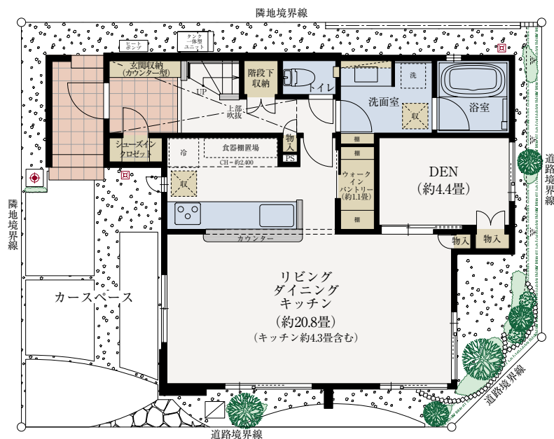
■1階平面図
