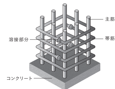
溶接閉鎖型せん断補強筋概念図
