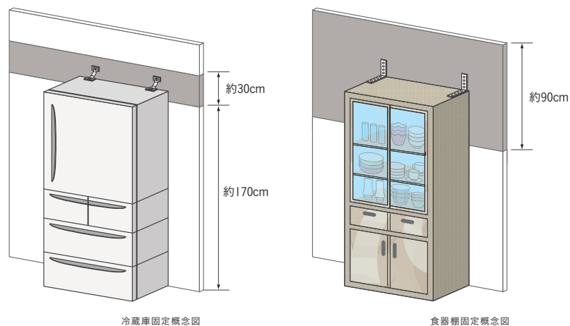
冷蔵庫固定概念図
