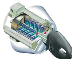
ディンプルシリンダー概念図
