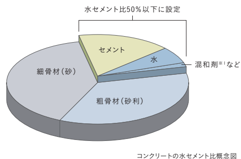
コンクリートの水セメント比概念図
