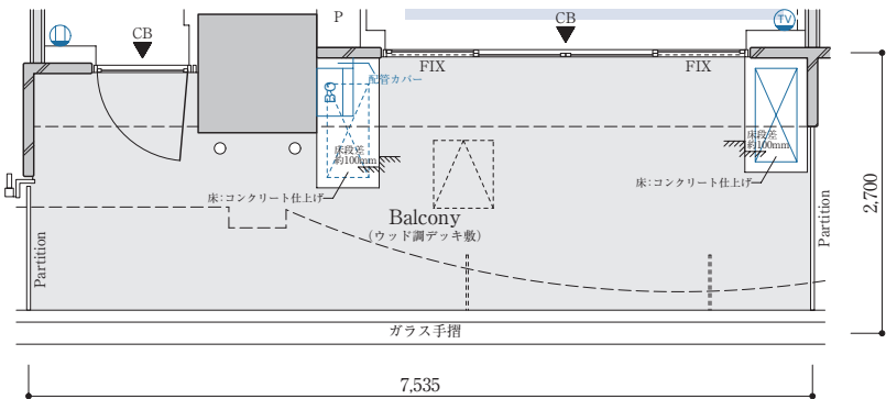
【4階部分図】
