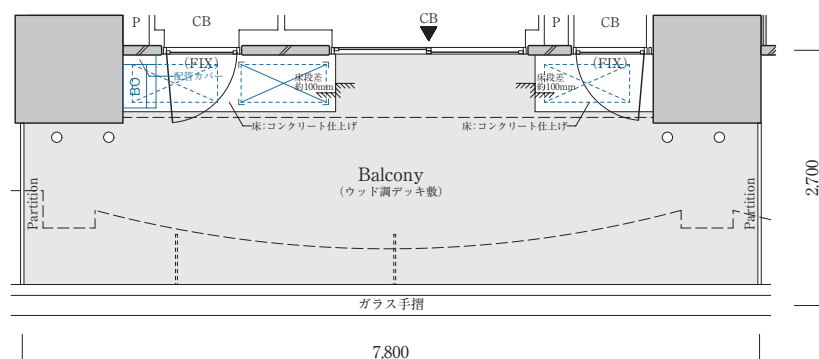
【4階部分図】
