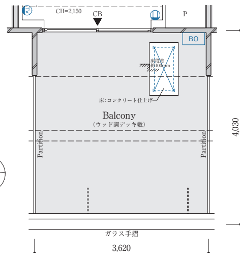
【4階部分図】
