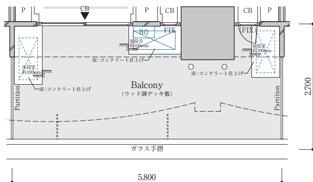
【4階部分図】
