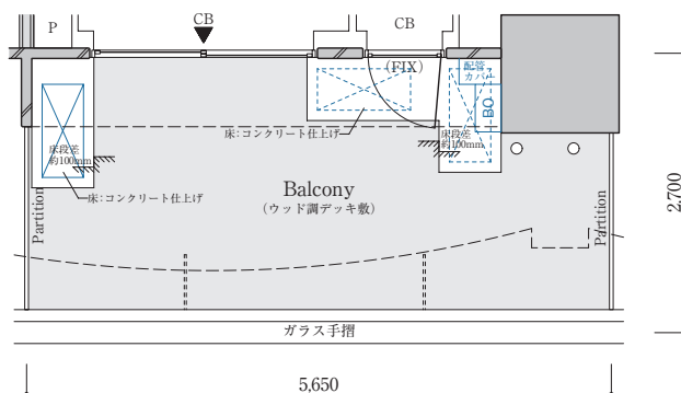
【4階部分図】
