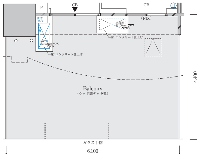
【4階部分図】
