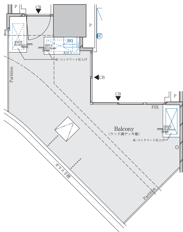
【4階部分図】
