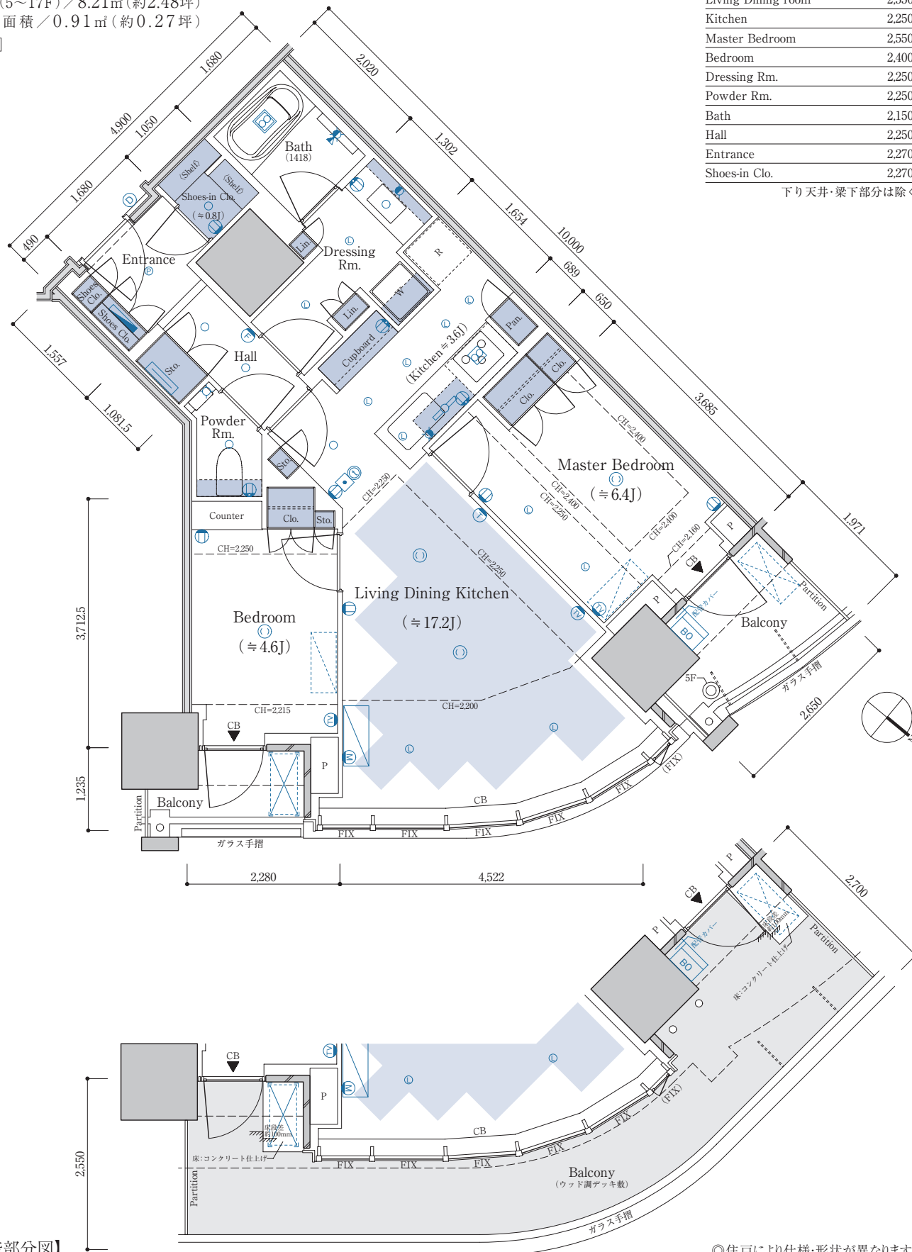
【4階部分図】
