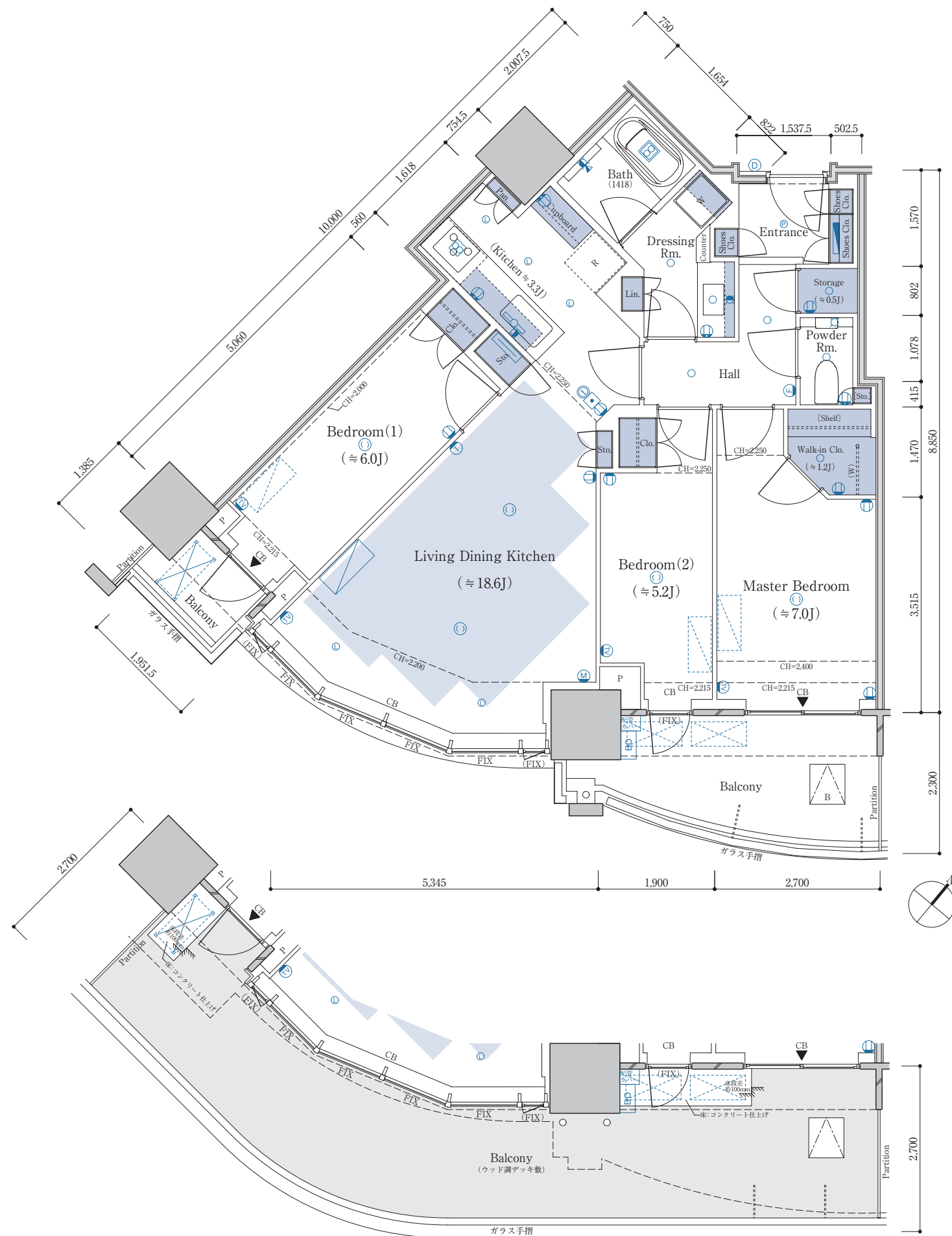
【4階部分図】
