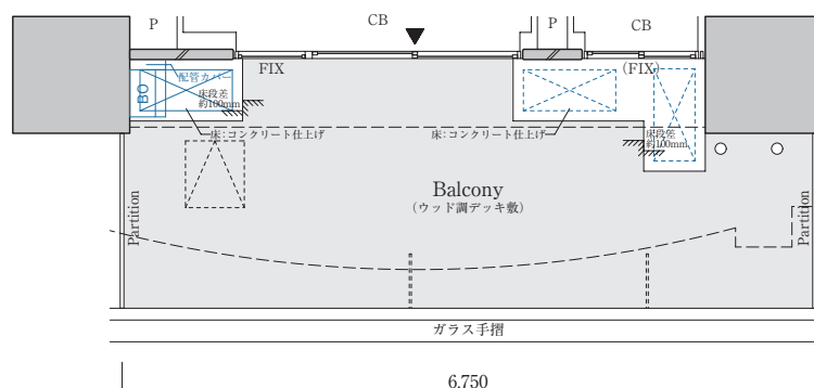
【4階部分図】
