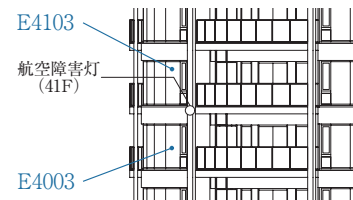
航空障害灯設置位置 西側立面拡大図 scale=約1/400
